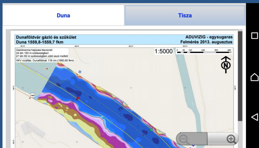
Dunai gázló helyszínrajz
